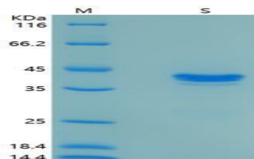
SDS-PAGE Result
